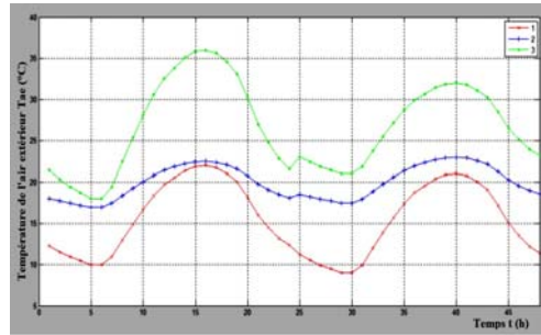
Fig. 2: Evolution de la température extérieure dans les trois cas et selon les deux jours consécutifs
