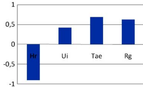
Fig. 10: Indice de sensibilité de la vitesse à phase constante par rapport aux entrées du modèle
