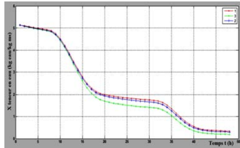
Fig. 3: Evolution de la teneur en eau dans les trois cas et selon les deux jours consécutifs
