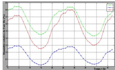
Fig. 6: Evolution de l'humidité relative pour les jours consécutifs, pour les trois cas
