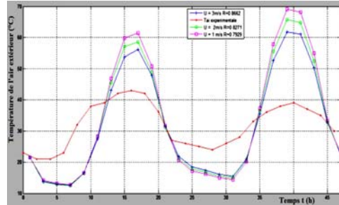
Fig. 12: Evolution de la température de l'air intérieur expérimentale et simulée
