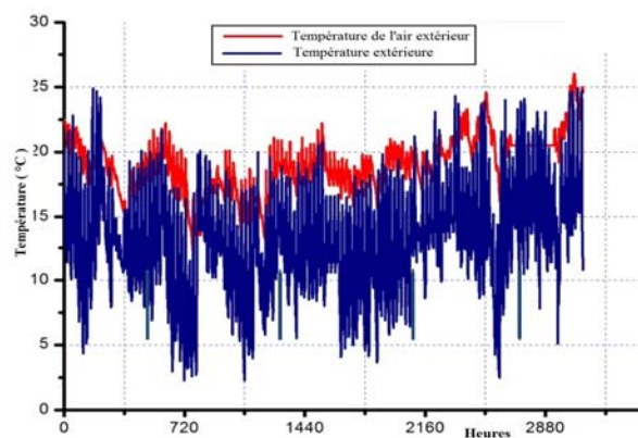
Fig. 5: Evolution de la température de l'air intérieur de la cellule étudiée et de la température extérieure
