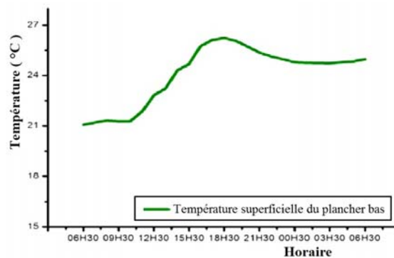
Fig. 7: Evolution de la température superficielle du plancher bas
