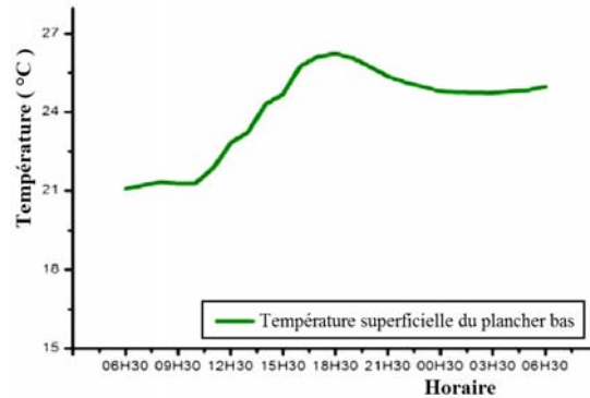
Fig. 8: Evolution de la température superficielle de la dalle (pendant 24h, décembre)
