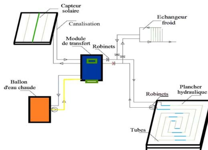
Fig. 1: Schéma de description du dispositif
