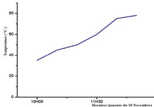
Fig. 4: Evolution de la température du fluide caloporteur au niveau du capteur solaire
