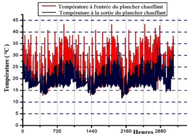
Fig. 6: Evolution de la température à l'entrée et à la sortie du plancher chauffant
