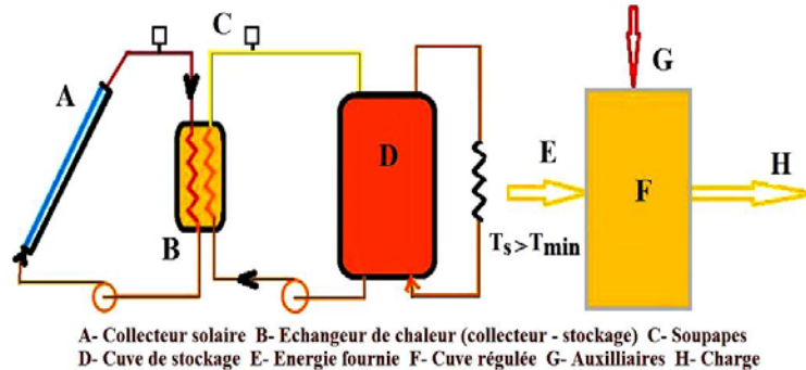
Fig. 2: Configuration standard d'un système de chauffe eau solaire fonctionnant en boucle fermée et sur laquelle est basée la méthode f -Chart [20]
