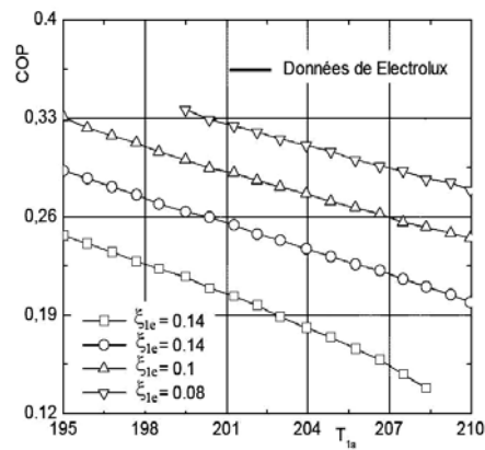
Fig. 6: variation de COP= ( T_{1a} , \xi_{1e} ), pour le cycle CAD-1 (concentration de la solution riche 0.35)
