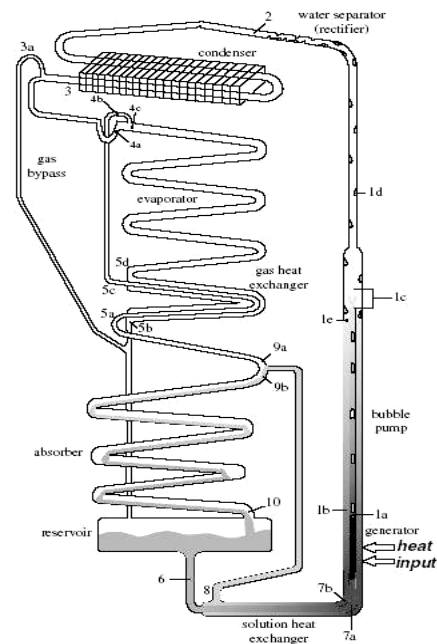
Fig. 2: Cycle à absorption-diffusion CAD-2 \text{NH}_3\text{-H}_2\text{O-H}_2 (adopté par Zohar et al. [10])
