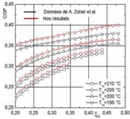
Fig. 7: Variation de COP = (\xi_6, T_{1a}) , pour le cycle CAD-2 (concentration de la solution pauvre 0.1)
