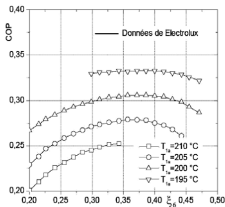
Fig. 5: Variation de COP = ( \xi_6 , T_{1a} ), pour le cycle CAD-1 (concentration de la solution pauvre 0.1)
