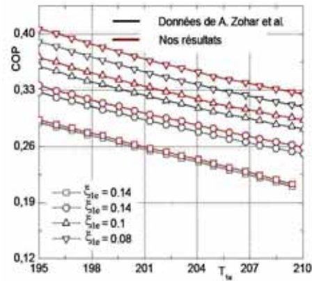
Fig. 8: Variation de COP = (T_{1a}, \xi_{1e}) , pour le cycle CAD-2 (concentration de la solution riche 0.35)
