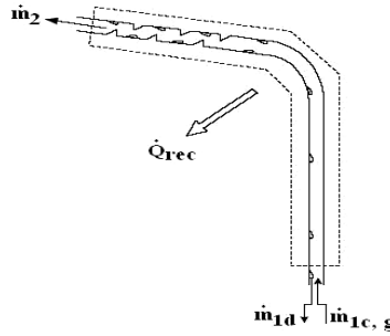
Fig. 3: Volume de contrôle du rectificateur
