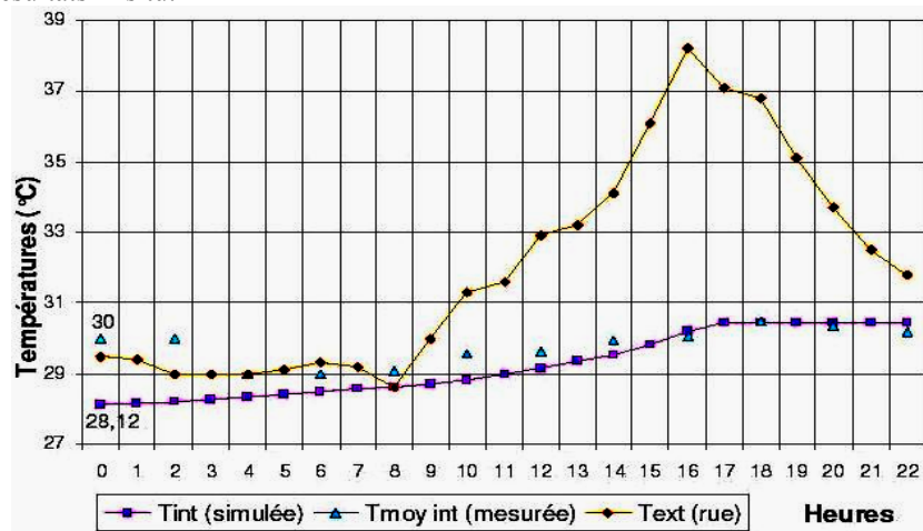
Fig. 24: Comparaison entre les températures moyennes intérieures et extérieures mesurées et les températures intérieures simulées (R.D.C.)
