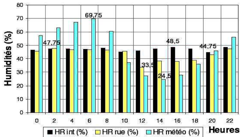
Fig. 15: Variation de l'humidité relative moyenne intérieure et extérieure (R.D.C.)
