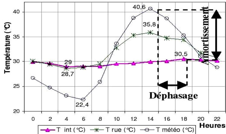
Fig. 9: Variation de la température moyenne intérieure et extérieure (R.D.C)
