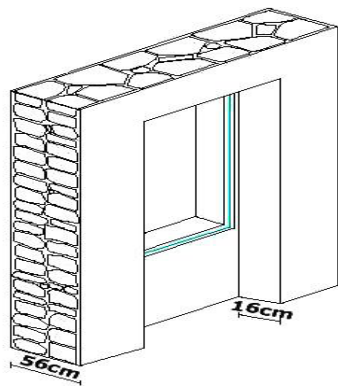
Fig. 10: Epaisseur du mur externe
