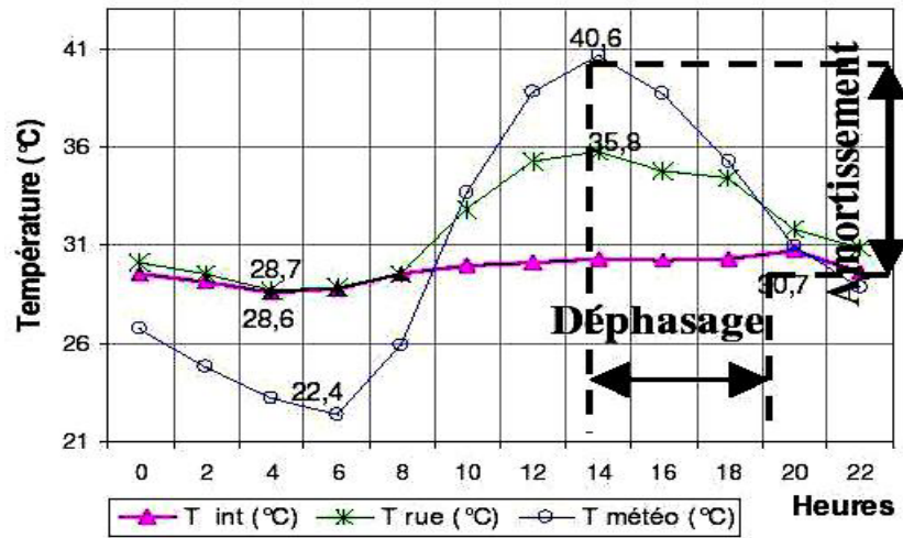
Fig. 16: Variation horaire de la température moyenne intérieure et extérieure (étage)
