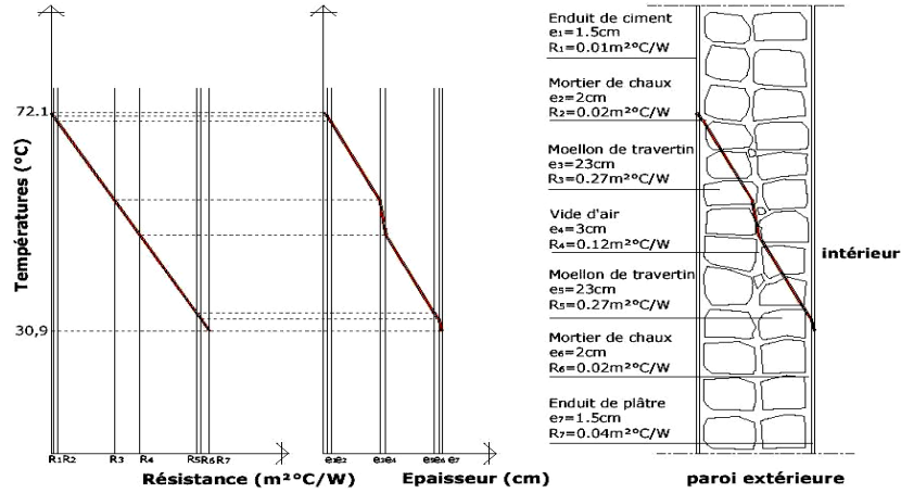
Fig. 14: Tracé du gradient thermique
