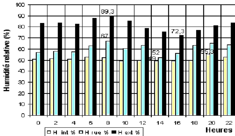
Fig. 19: Variation de l'humidité relative (R.D.C)
