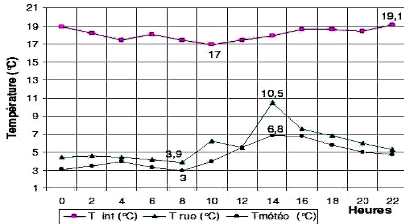
Fig. 18: Variation horaire de la température moyenne intérieure et extérieure (R.D.C.)
