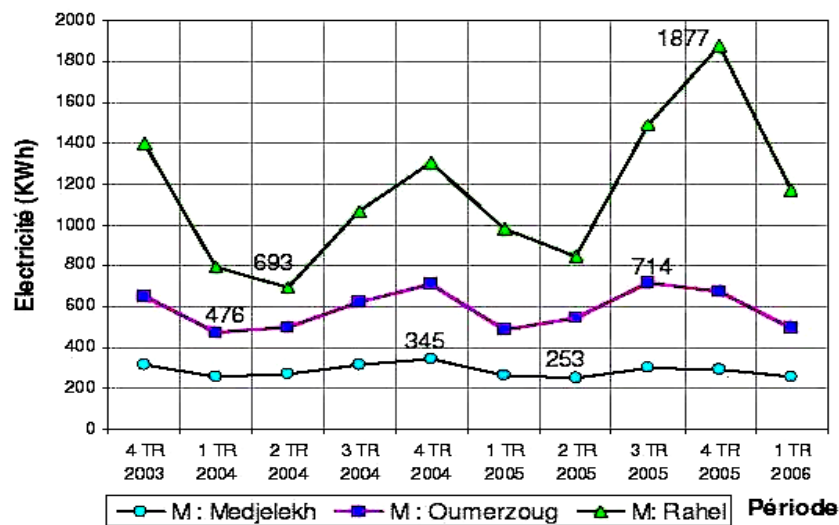
Fig. 20: Consommation de l'électricité des trois maisons sur une période de dix trimestres
