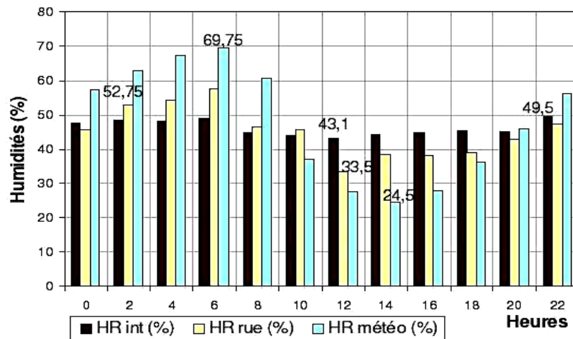
Fig. 17: Variation de l'humidité moyenne intérieure et extérieure (Etage)
