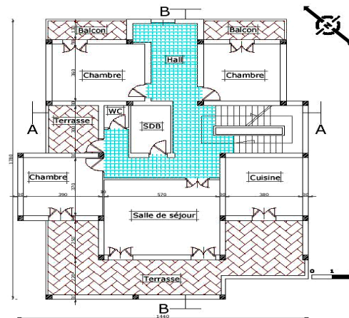
Fig. 8: Plan étage de la villa ( source auteur )
