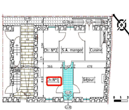
Fig. 3: Plan RDC (source auteur)
