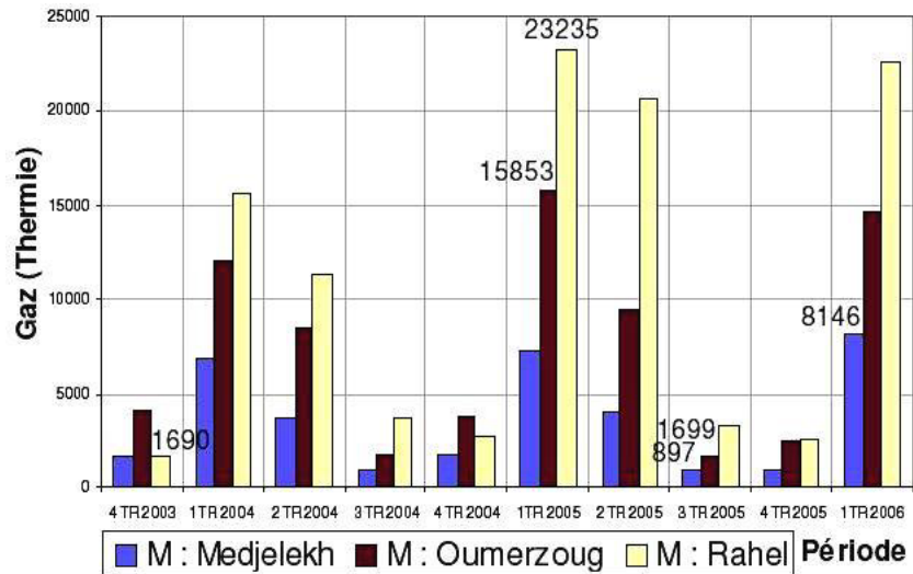
Fig. 23: Consommation du gaz des trois maisons sur une période de dix trimestres
