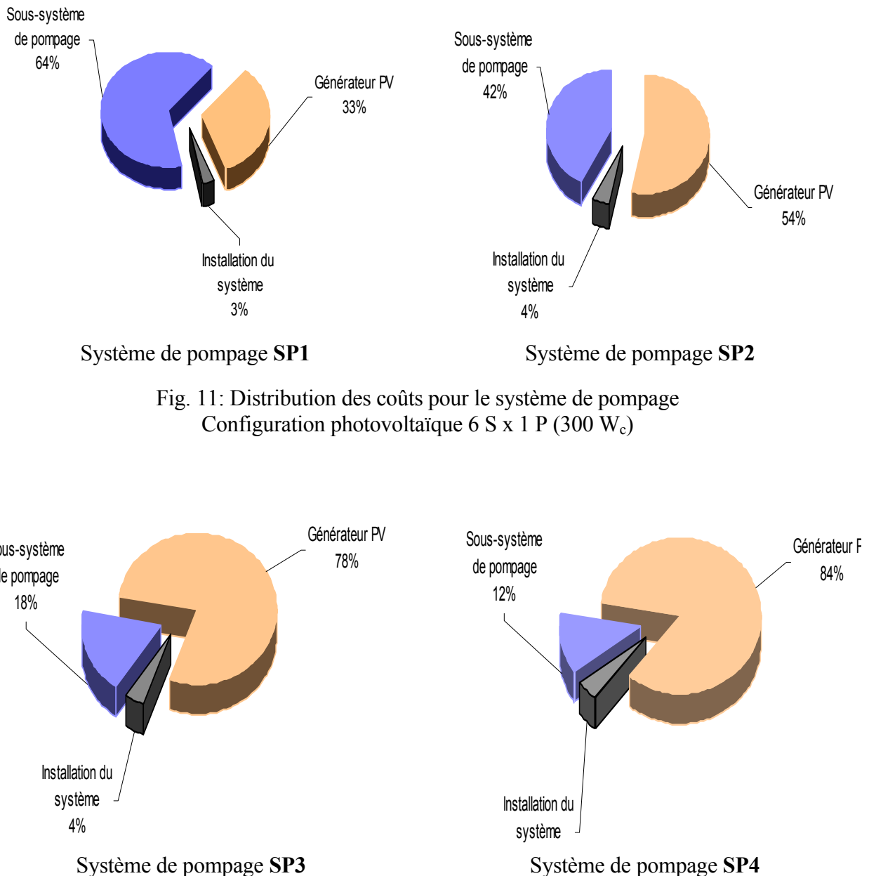
Fig. 12: Distribution des coûts pour le système de pompage Configuration photovoltaïque 7 S x 4 P (1400 W c )
