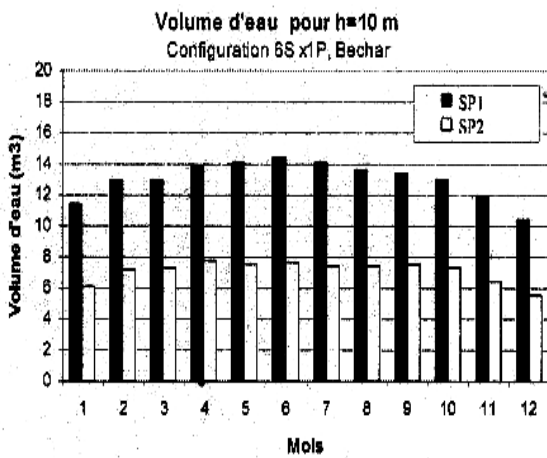
Fig. 5: Volume d'eau pompé mensuel h = 10 m
