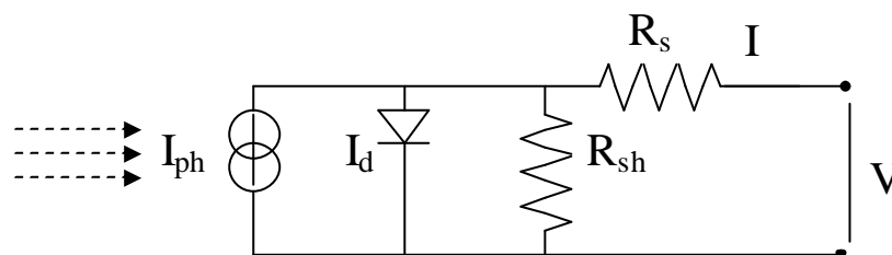
Fig. 4 - Schéma équivalent déduit de l'équation (5) à une exponentielle (SEM) associé
