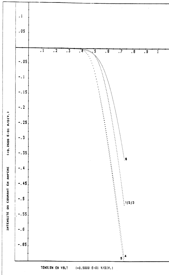
Fig. 9: Cas d'une photopile de qualité médiocre ( R_{sh} de 40 Ohm) sous faible éclaircissement 0,2 \times AM1 . Comparaison de la mesure (1) avec les courbes reconstituées à partir des déterminations de paramètres effectuées par résolution numérique SEM (2) et VDEM (3), et à l'aide des méthodes approximatives de [80WAR.U.] (4), [Singal 1981] (5), [Araujo et Sanchez 1982] (6), et la combinaison des méthodes [Wolf et Rauschenbach 1963, et Panayotatos et Card 1978] pour la courbe (7).
