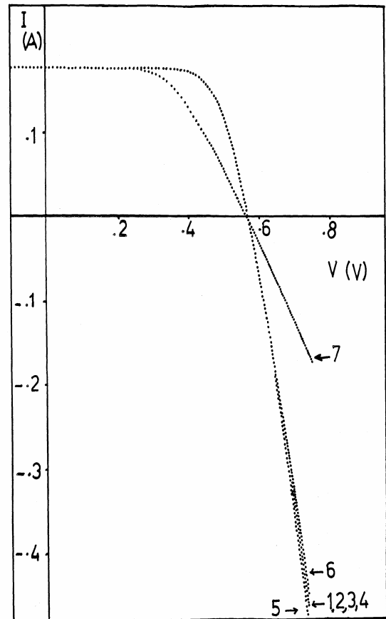
Fig. 10 : Cas d'une photopile de qualité médiocre ( R_{sh} de 40 Ohm) sous éclaircissement AM0. Comparaison de la mesure (1) avec les courbes reconstituées à partir des déterminations de paramètres effectuées par résolution numérique SEM (2) et VDEM (3), et à l'aide des méthodes approximatives de [Kammer et Ludington 1977] (4), [Singal 1981] (5), et [Araujo et Sanchez 1982] (6).
