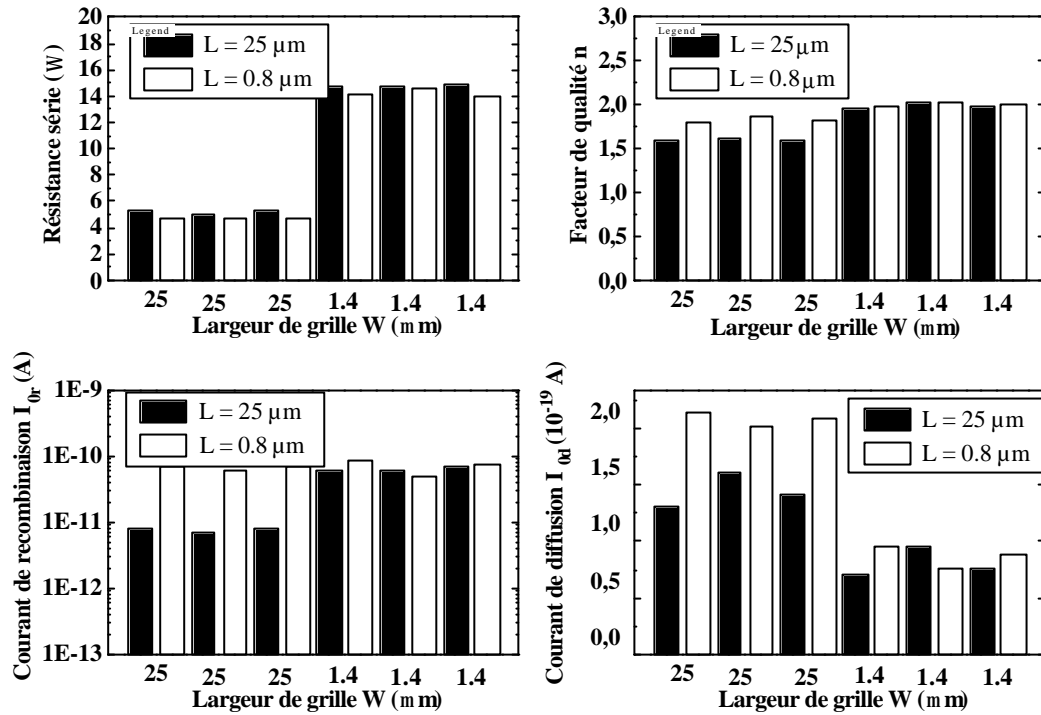
Fig. 13 - Variations des paramètres de la jonction en fonction des dimensions de la grille (W/L).
