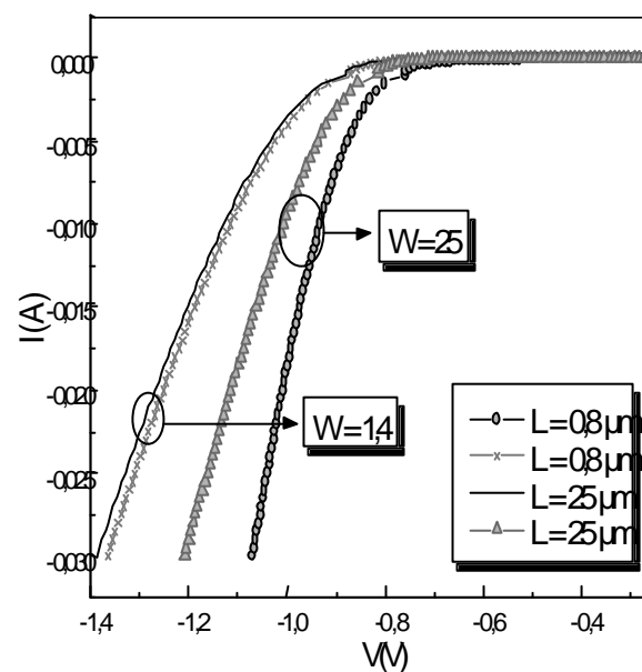
Fig. 12 - Caractéristiques I(V) de jonctions drain-substrat pour des transistors de même longueur de canal ( L ) illustrant l'influence importante de la valeur de la largeur ( W ) du canal.
