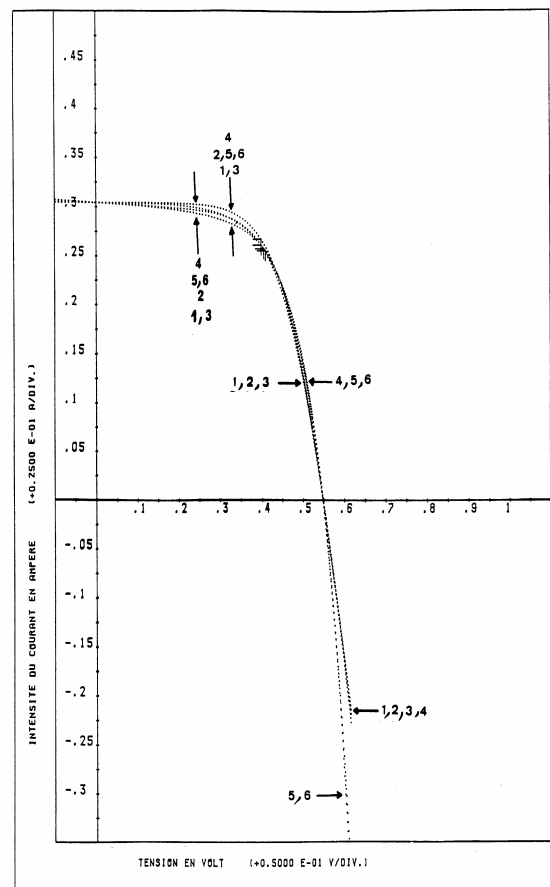
Fig. 8 : Cas d'une photopile de bonne qualité ( R_{sh} de 2000 Ohm) sous fort éclaircissement 1,3xAM1 . Comparaison de la mesure (1) avec les courbes reconstituées à partir des déterminations de paramètres effectuées par résolution numérique SEM (2) et VDEM (3), et à l'aide des méthodes approximatives de [Warashina et Ushirokawa 1980] (4), [Singal 1981] (5), [Araujo et Sanchez 1982] (6), et la combinaison des méthodes [Wolf et Rauschenbach 1963, et Panayotatos et Card 1978] pour la courbe (7).
