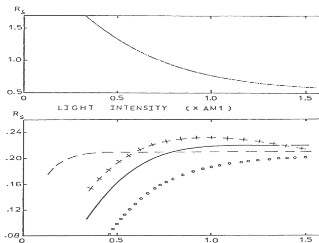
Fig. 6 - Variations de la résistance série en fonction de l'éclairement obtenues à partir des méthodes proposées par: [Cape et Zehr 1980] en petit pointillé représentée dans le cadre supérieur et [Singal 1981] ligne de croix, [Warashina et Ushirokawa 1980.] ligne de traits, [Araujo et Sanchez 1982] ligne de ronds, et la ligne pleine obtenue par résolution numérique du SEM, dans le cadre inférieur.
