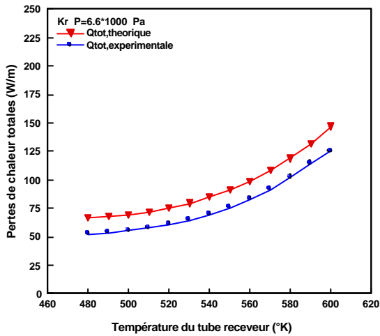
Fig. 12 : Caractéristique des pertes thermiques d'un tube absorbeur utilisant le krypton dans l'espace annulaire ( P=6.6 \times 10^3 Pa)
