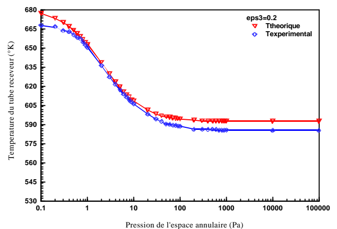
Fig.3 : Variation de la température de l'absorbeur ( \epsilon = 0.2 ) en atmosphère raréfiée ( \epsilon = 0.3 )
