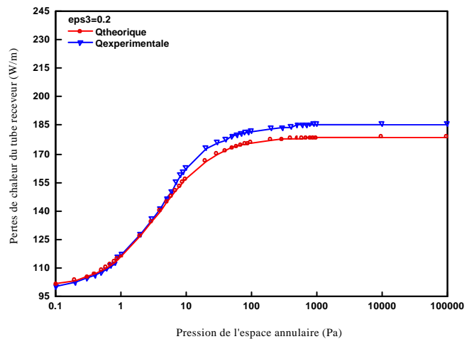
Fig.5 : Effets de la pression sur les pertes du tube absorbeur ( T_i = 589 °K, \epsilon = 0.2 )
