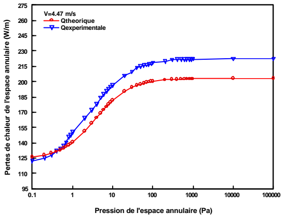
Fig. 8 : Effets du vent sur les pertes thermiques ( T_i = 589^\circ\text{K} , \epsilon = 0.25 , V = 4.47 m/s )
