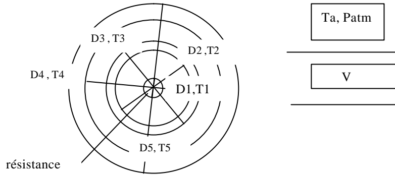
Fig.1 : coupe du tube absorbeur
