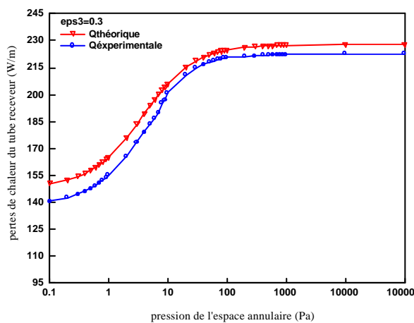
Fig.4 : Effets de la pression sur les pertes du tube absorbeur ( T_i = 589 °K, \epsilon = 0.3 )
