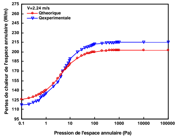
Fig.7 : Effets du vent sur les pertes thermiques ( T_i = 589^\circ\text{K} , \epsilon = 0.25 , V = 2.24 m/s )
