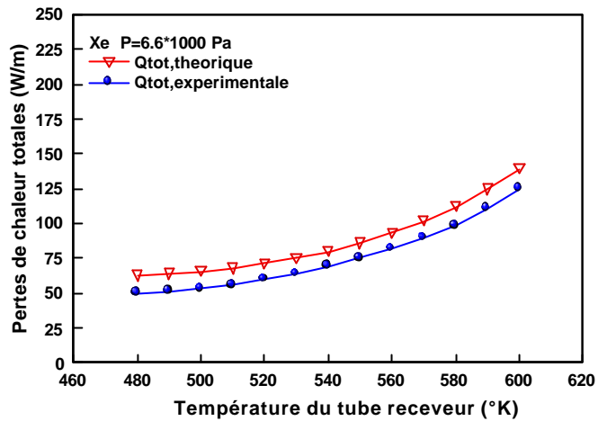
Fig. 13 : Caractéristique des pertes thermiques d'un tube absorbeur utilisant le xénon comme fluide annulaire ( P=6.6 \times 10^3 Pa)
