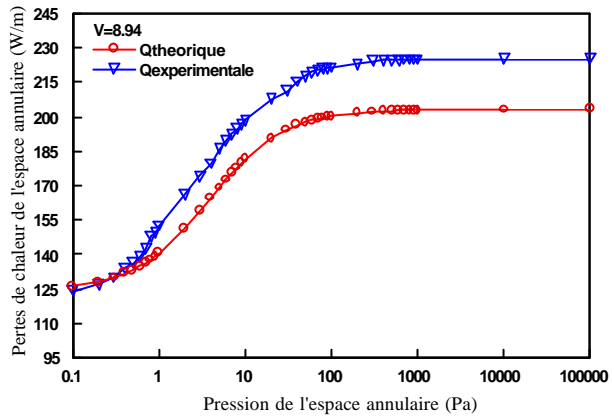
Fig.9 : Effets du vent sur les pertes thermiques ( T_i = 589^\circ\text{K} , \epsilon = 0.25 , V = 8.84 m/s )
