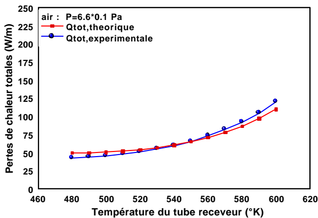
Fig.10 : Caractéristique des pertes thermiques d'un tube absorbeur utilisant l'air comme fluide annulaire ( P = 6.6 \times 10^3 Pa )
