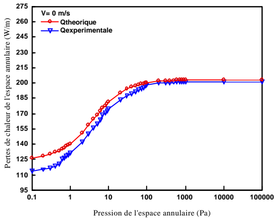
Fig.6 : Effets du vent sur les pertes thermiques ( T_i = 589^\circ\text{K} , \epsilon = 0.25 , V = 0 m/s )
