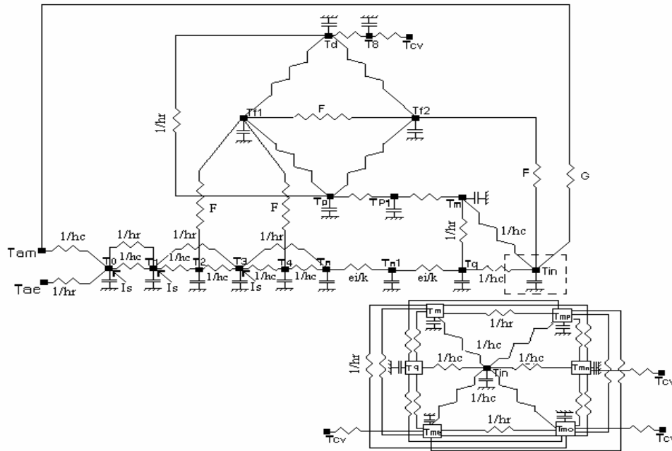
Fig. 2 : Schéma électrique.
