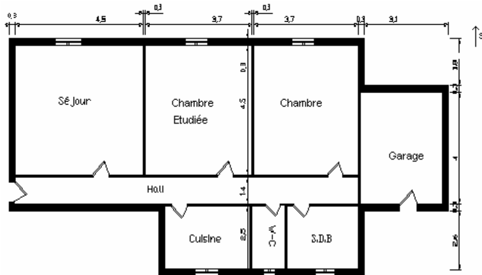
Fig. 4 : Plan R.d.C d'une habitation type.
