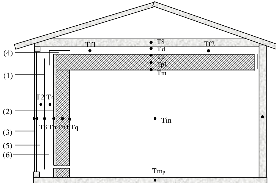
Fig. 1 : Modélisation du local.
