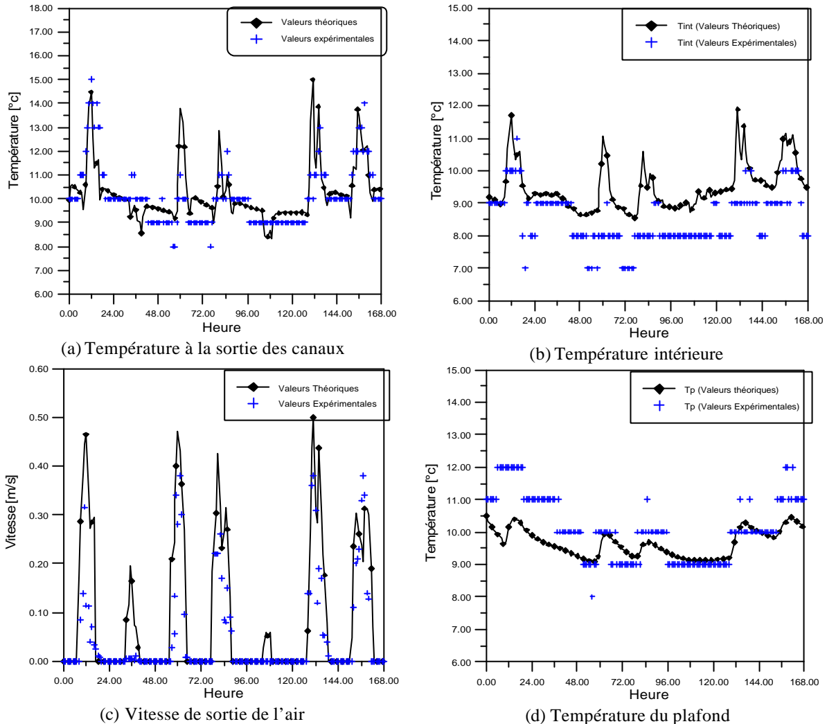
Fig. 3.1 : Confrontation des résultats théoriques et expérimentaux.
