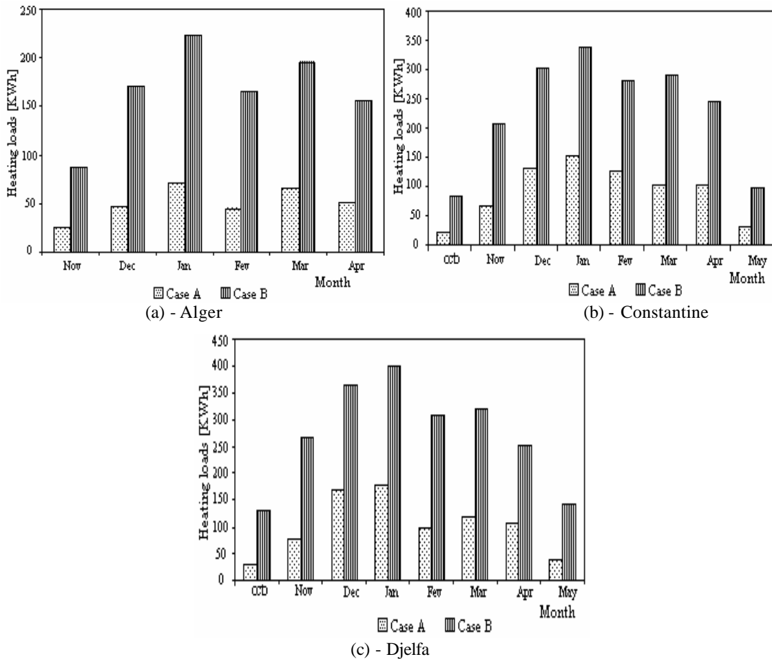
Fig. 7 : Besoins mensuels de chauffage.
