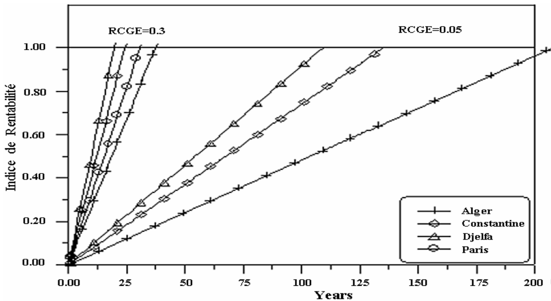
Fig. 8 : Indice de Rentabilité du système.
