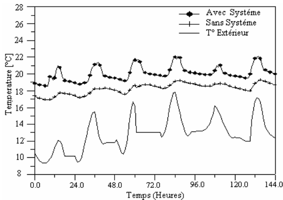
Fig. 5 : Température intérieure.
