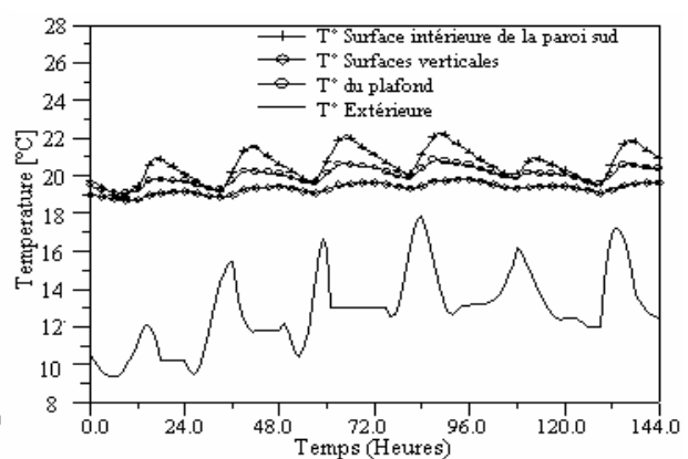
Fig. 6 : Température des parois.
